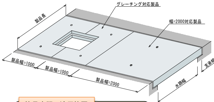
簡易床版の適用範囲
