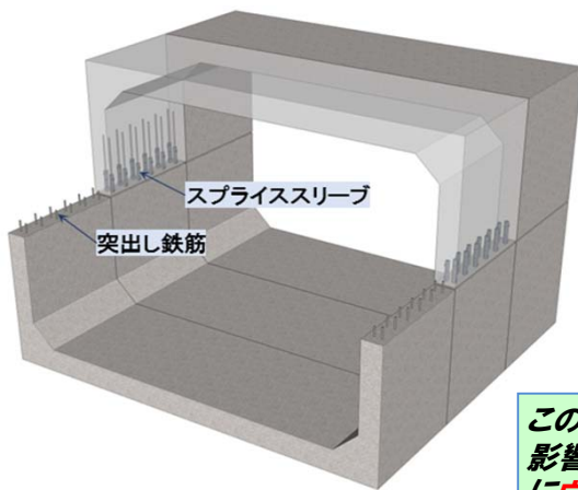
スプライススリーブ概要図
