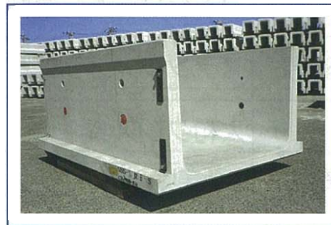
No.421 SSS-Ⅲ型フリーム (浮力対策対応型)
