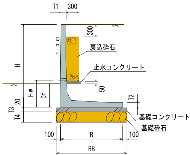
●HDウォール II型 標準断面寸法表
