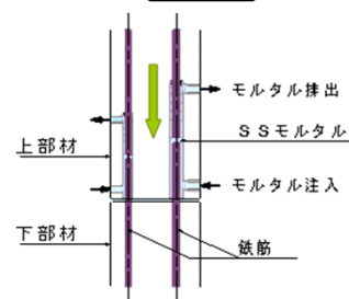
接手部
