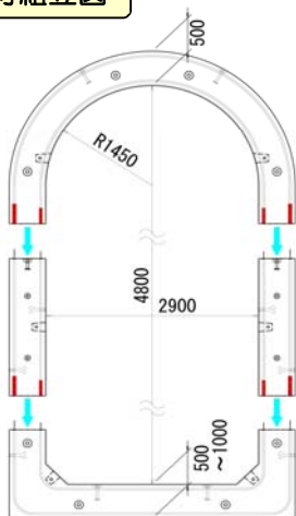
部材組立図
