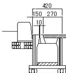
参考断面図
