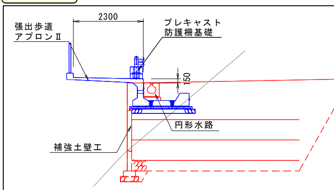
参考断面図
