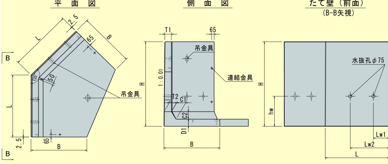
規格図
